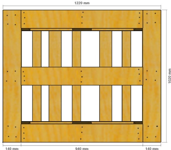
VISTA INFERIOR
