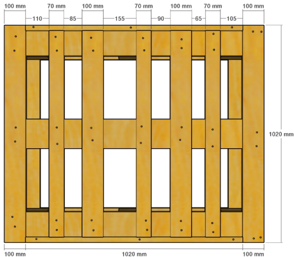
VISTA INFERIOR
