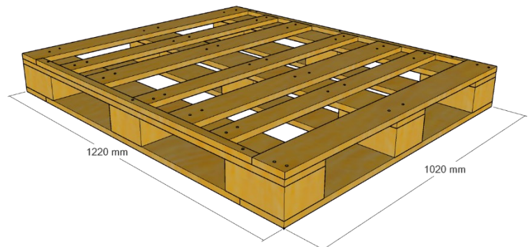
VISTA ISOMETRICA
